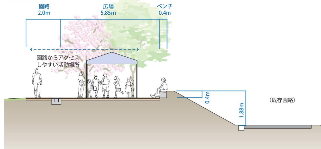
■A-A' 断面図
