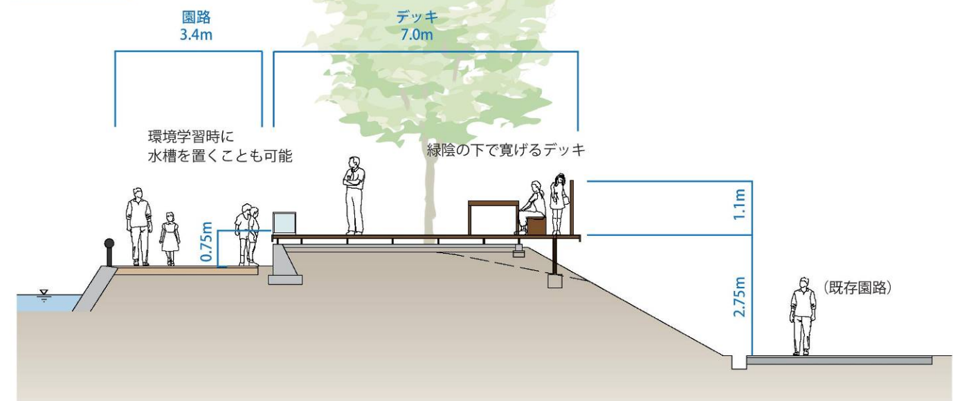
■B-B' 断面図
